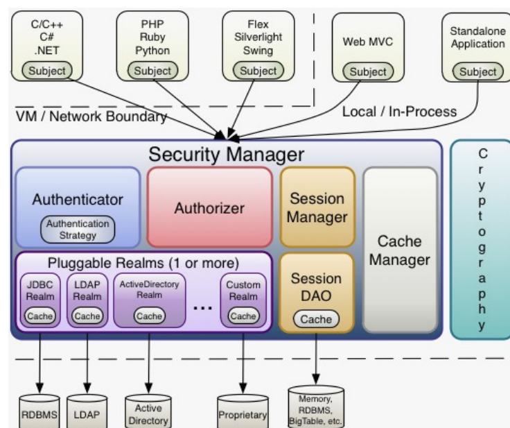
รูปที่ ๓ แผนภาพการรักษาความมั่นคงปลอดภัยสารสนเทศ
