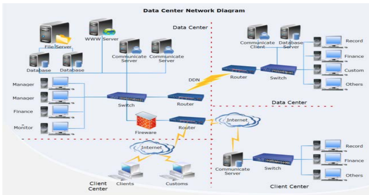
รูปที่ ๑ แผนผังการเชื่อมโยงเครือข่าย (Network diagram)
